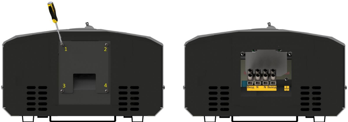
Рисунок 9. Схема снятия защитной крышки снизу корпуса стабилизатора
